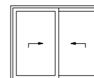
dvodelni element sa dva podizno-klizna krila
